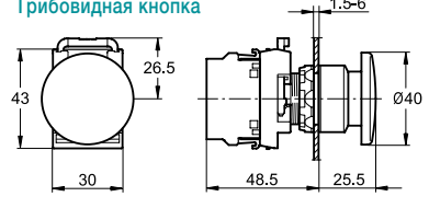
Грибовидная кнопка
