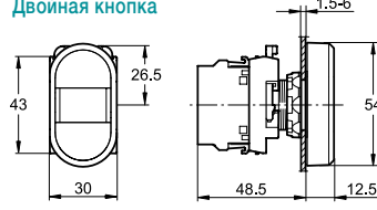
Двойная кнопка
