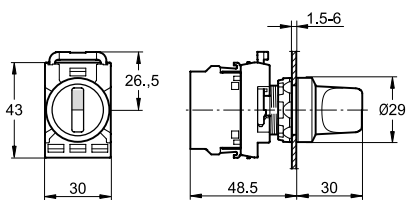
Переключатель
