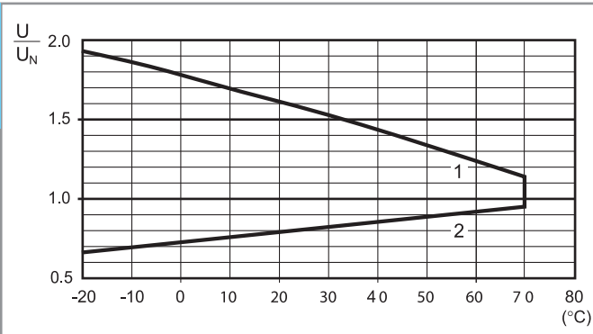
R 60 - Отношение рабочего диапазона для DC к температуре окр. среды
