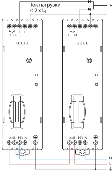
Параллельное подключение
