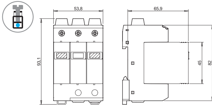
Тип 7P.26.9.000.1015 Винтовые клеммы
