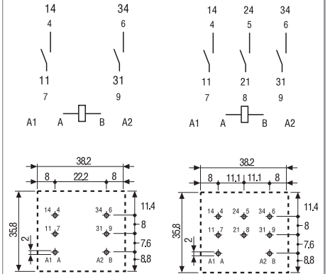
62.22 - 0300 62.23 - 0300 Вид со стороны выводов
