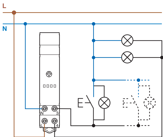
3-проводное соединение
