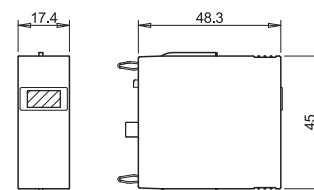
Тип 7P.10/20 Заменяемый модуль
