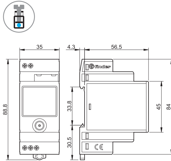
12.61 / 12.A1 Винтовые клеммы
