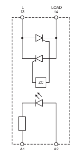
Упрощенная принципиальная схема
