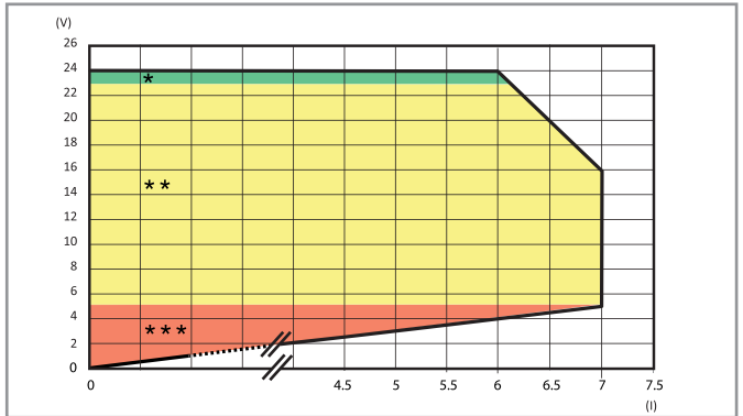
FB78-4 Выходное напряжение VS выходного тока (78.1D)
