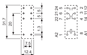
Вид со стороны выводов
