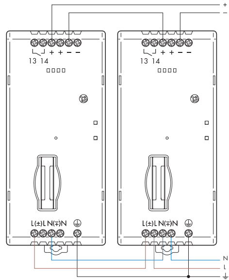
Последовательное подключение
