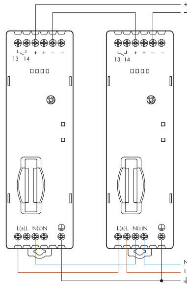
Последовательное подключение
