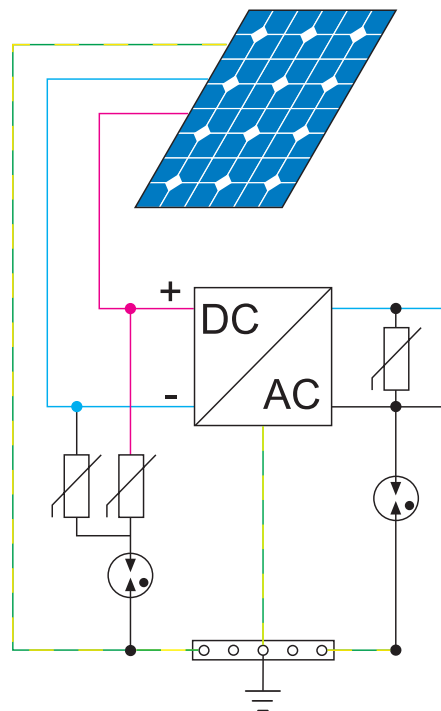
Рис 10: пример фотогальванической системы для здания не оборудованного системой защиты от молнии; защита со стороны DC при помощи УЗИП с U_{oc\ stc} = 420\ В , и защита со стороны AC устройством 7P.22, характерным для систем TT.
