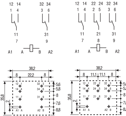
62.22 62.23 Вид со стороны выводов
