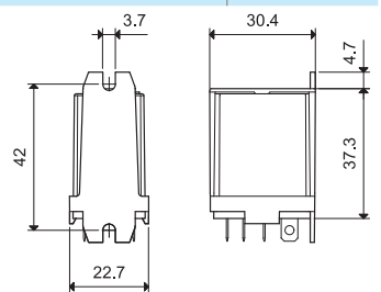
056.26 с реле
