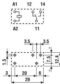
Вид со стороны выводов
