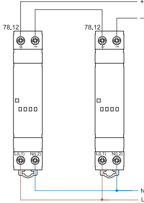
последовательное соединение
