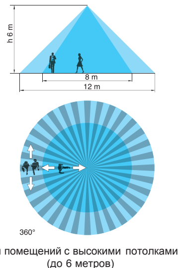
18.31...0031 - Монтаж в помещениях с высокими потолками
