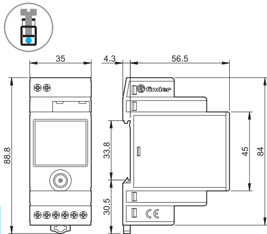
12.62 / 12.A2 Винтовые клеммы
