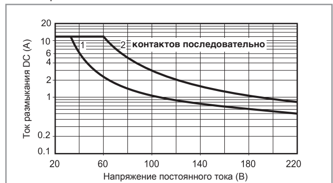
H 56 - Макс. отключающая способность DC1 Версия с NO контактом
