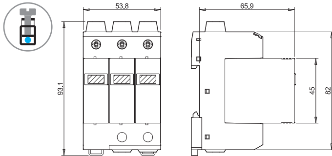
Тип 7P.23.9 Винтовые клеммы
