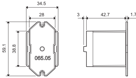
Фланцевый адаптер крепления для реле типов 65.31.xxxx.xxx9
