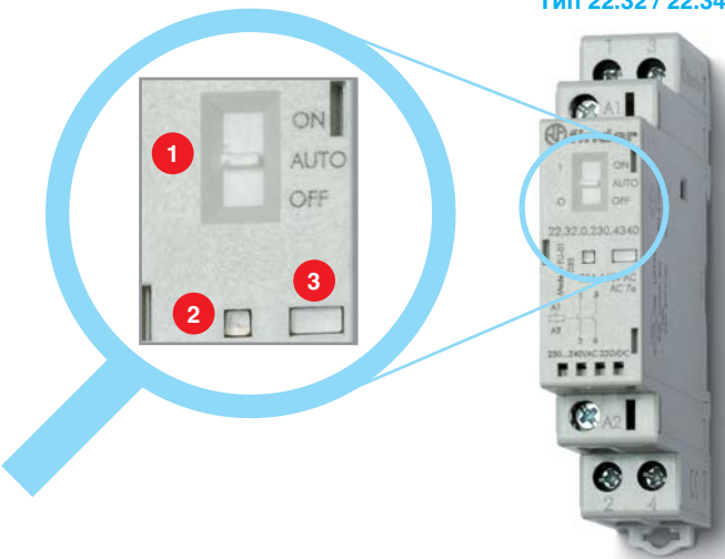
Тип 22.32 / 22.34
