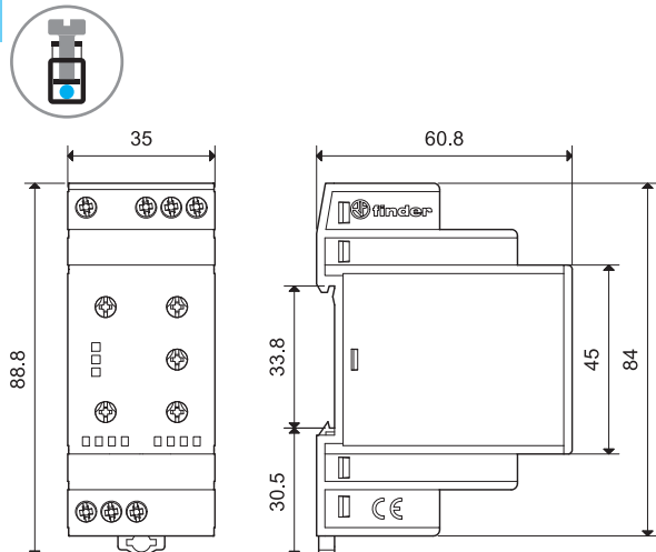
70.61 Винтовые клеммы
