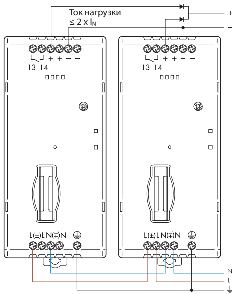
Параллельное подключение
