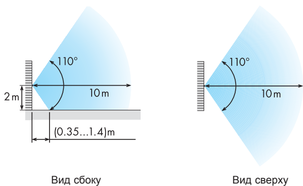
18.01, 18.11 - Настенный монтаж
