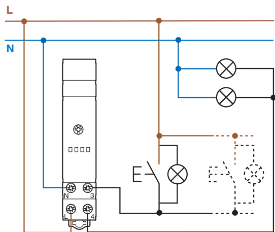
4-проводное соединение
