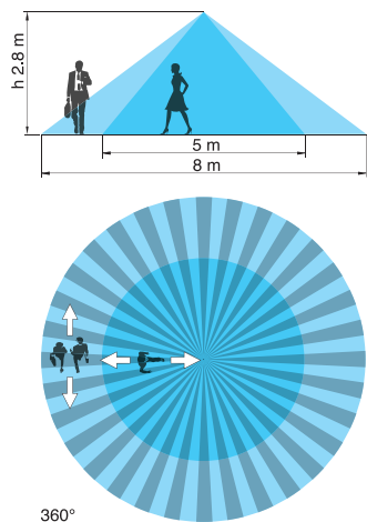
18.21, 18.31 - Монтаж на потолке
