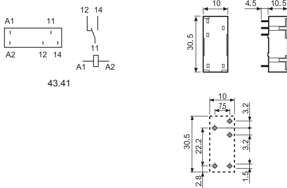
Вид со стороны выводов
