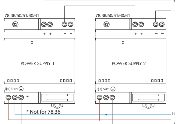
последовательное соединение
