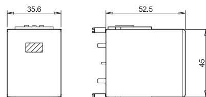
Тип 7P.00 Заменяемый модуль
