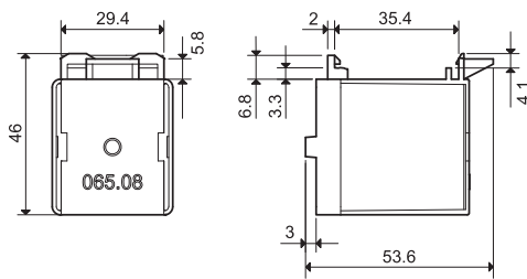
Адаптер 35 мм рейки (EN 60715) для реле типов 65.31.xxxx.xxx9
