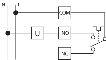
Схема подключения
