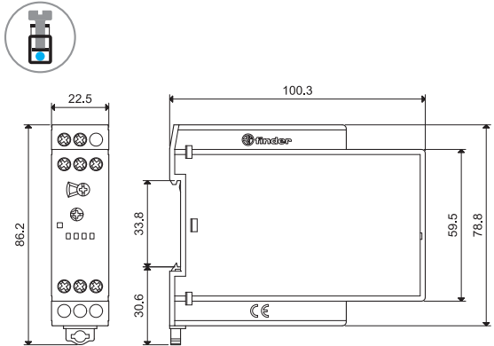
83.62 Винтовые клеммы
