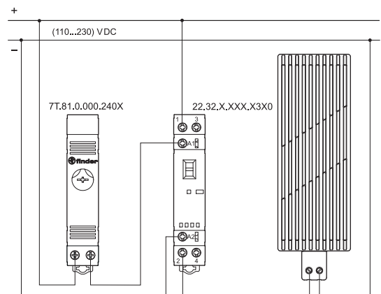
Версия для DC
