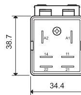
Адаптер 35 мм рейки (EN 60715) для реле типов 65.31.xxxx.xxx9
