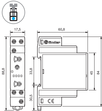
80.01 Винтовые клеммы
