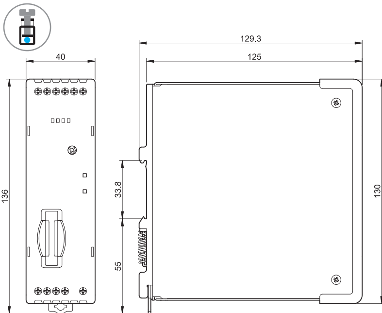
78.1C / 78.1D Винтовые клеммы
