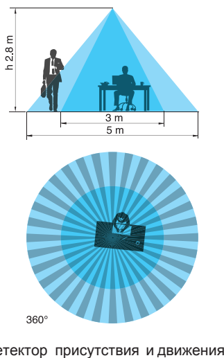
18.31...0031 - Монтаж на поверхности на потолке в помещении
