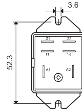
Фланцевый адаптер крепления для реле типов 65.31.xxxx.xxx9
