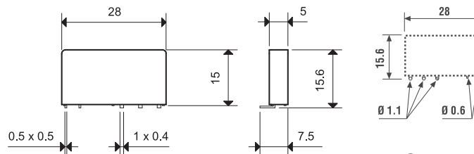
Вид со стороны выводов
