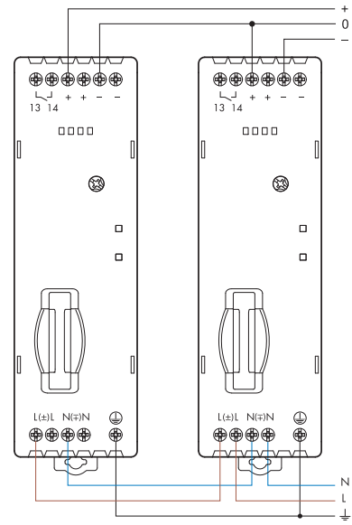
Сдвоенное подключение
