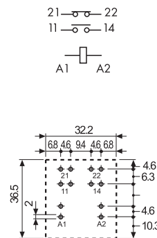
Вид со стороны выводов
