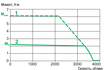
Серводвигатель BSH 070 2T С сервопреобразователем LXM 32●D30M2
