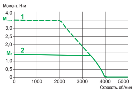
Серводвигатель BSH 070 1T С сервопреобразователем LXM 32●D18M2
