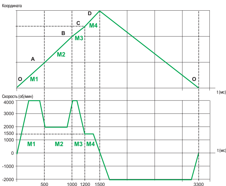
Пример перемещения, выполняемого за 5 шагов
