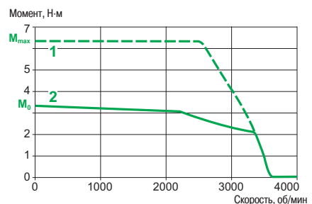
Серводвигатель BSH 100 1T С сервопреобразователем LXM 32●D30M2
