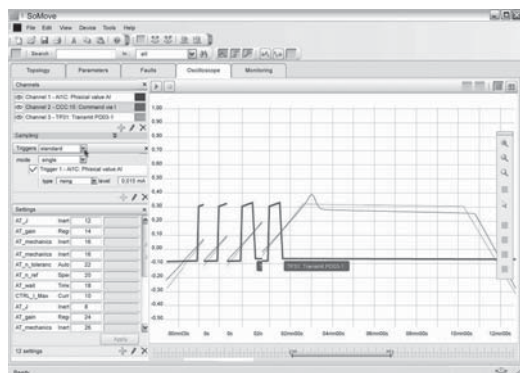
Оциллографирование при помощи ПО SoMove
