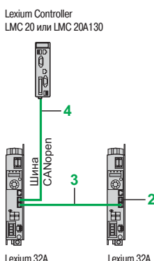
Пример архитектуры с управлением от контроллера перемещения LMC Lexium Controller
