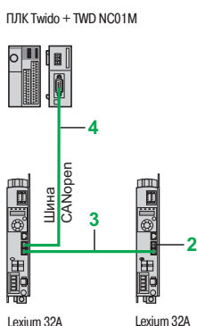
Пример архитектуры с управлением от ПЛК Twido
