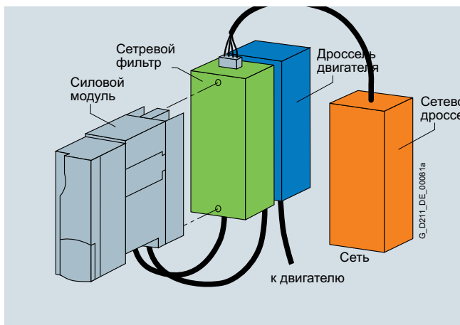
В случае более двух каркасных системных компонентов, к примеру, сетевой дроссель + дроссель двигателя + тормозной резистор, отдельные компоненты должны быть смонтированы сбоку рядом с силовым модулем PM340. При этом сетевой дроссель и дроссель двигателя должны быть расположены за силовым модулем, тормозной резистор сбоку рядом с ним.
