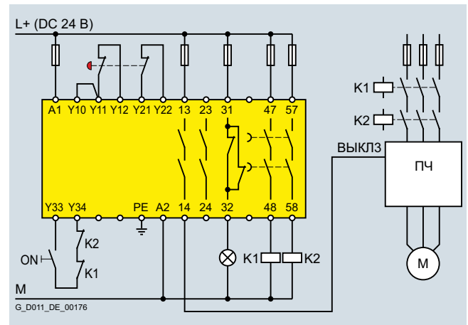
Обычное подключение
