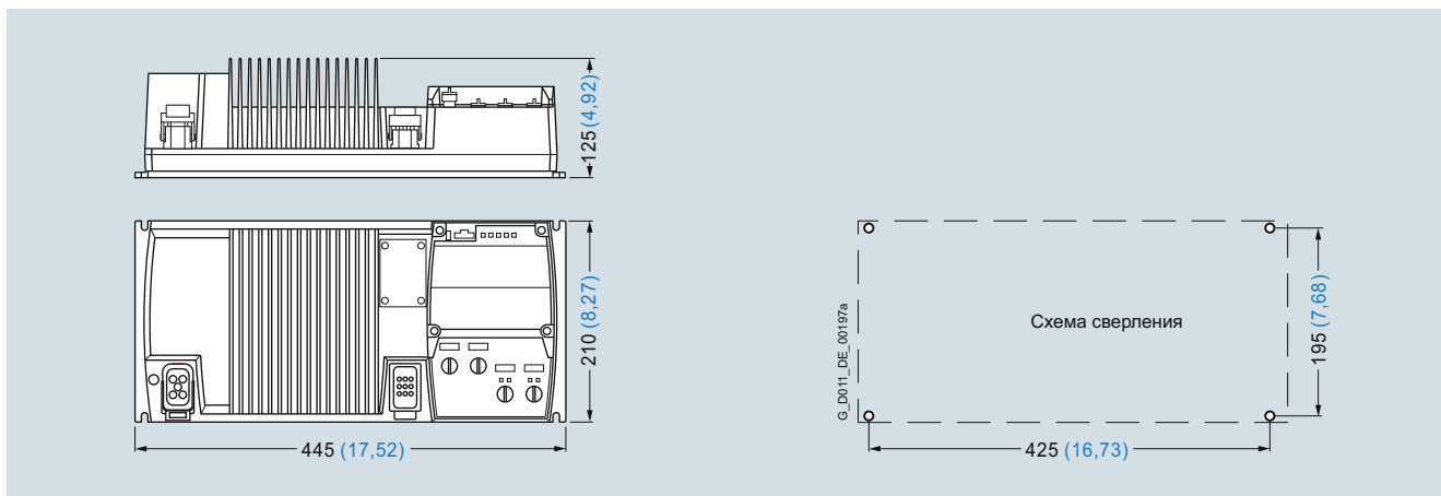
SINAMICS G110D типоразмер FSA со встроенным сетевым фильтром класса А
