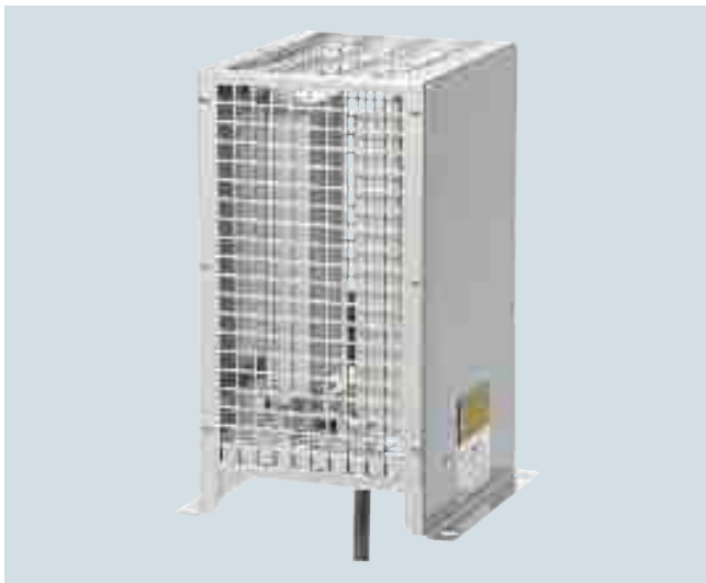
Тормозной резистор для силовых модулей PM240 типоразмер FS D
