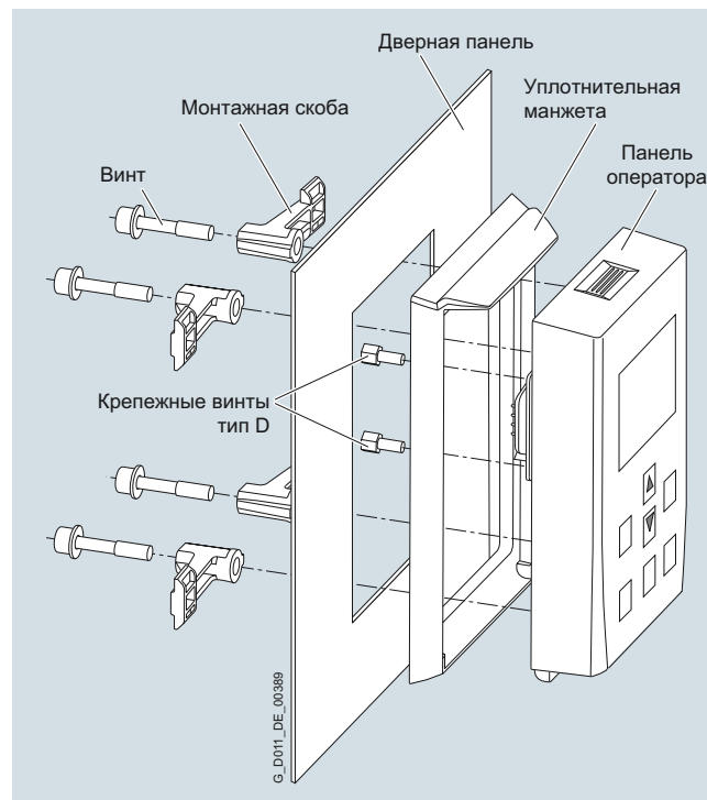
Набор для монтажа в дверцу со вставленной ВОР-2
