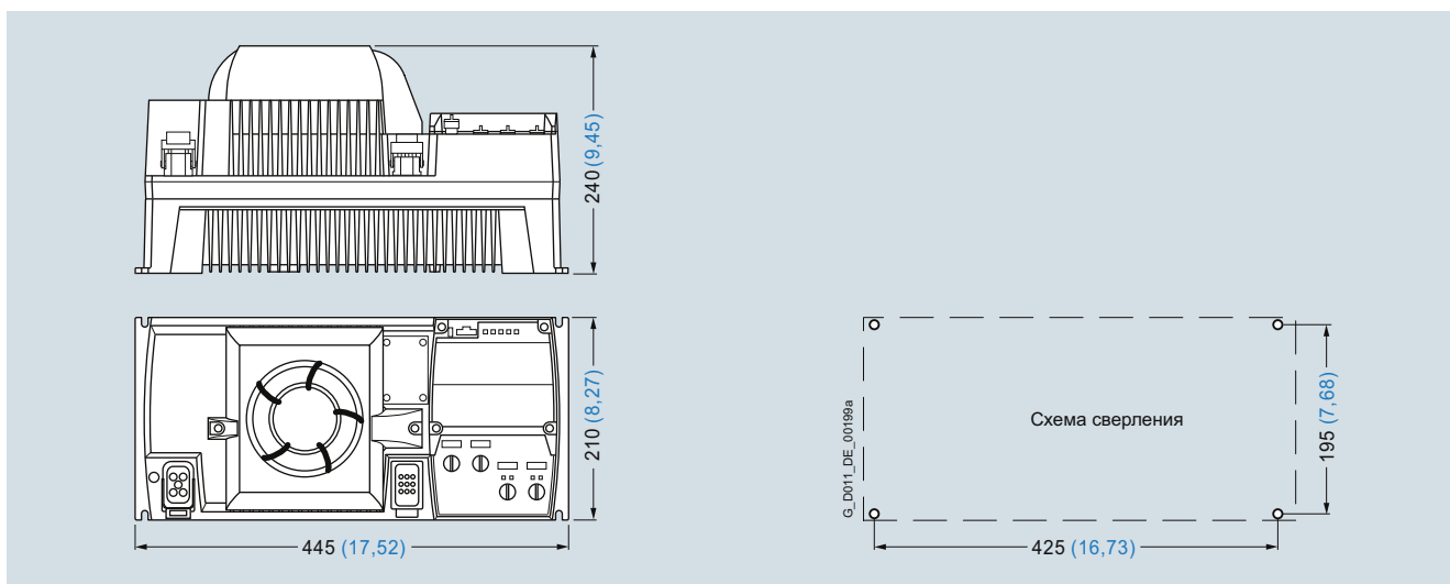
SINAMICS G110D типоразмер FSC со встроенным сетевым фильтром класса А
