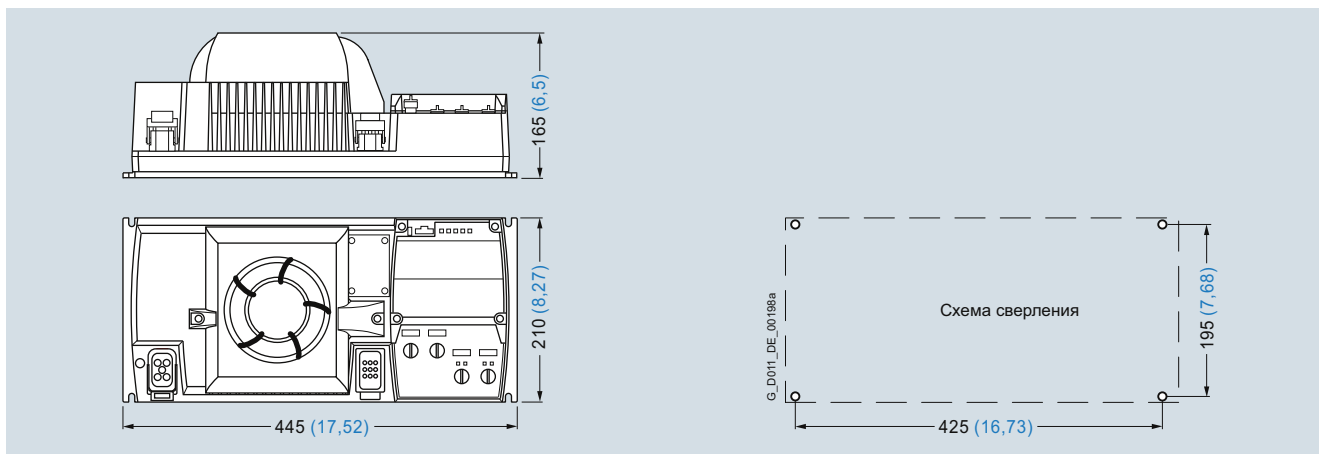
SINAMICS G110D типоразмер FSB со встроенным сетевым фильтром класса А
