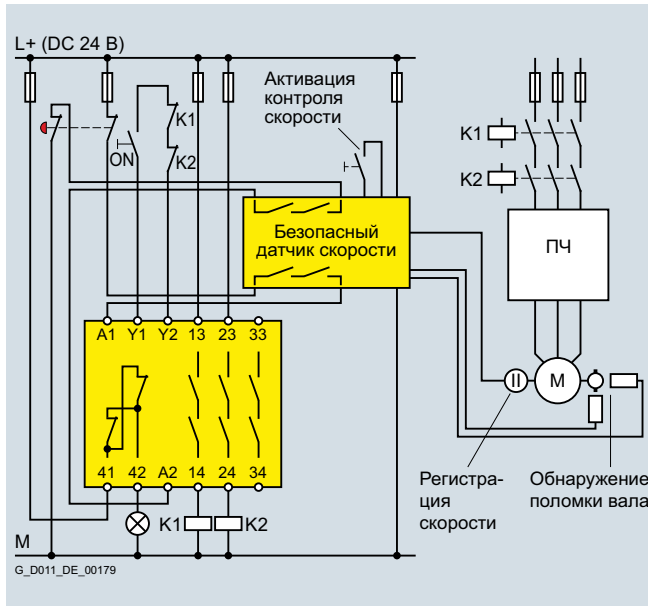
Обычное подключение
