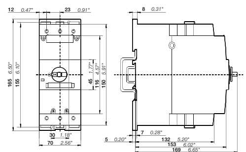
MO495, MO496
