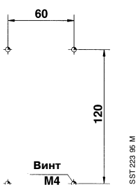
Схема отверстий DRB 6/DRB 7
