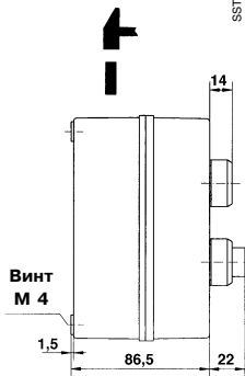
Габаритный чертеж DRB 6/DRB 7
