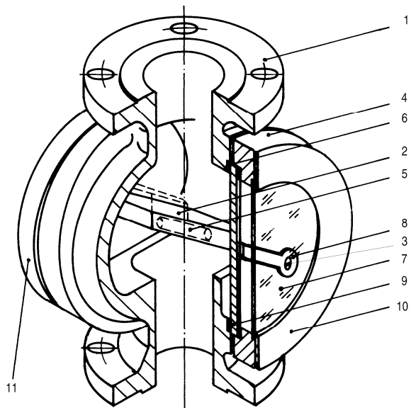
Рис. 2 Клапанный Индикатор Протока F I Прима д. непрозрачных жидк.
