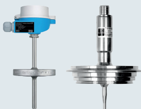
Термопреобразователи сопротивления Наиболее используемый тип контактных промышленных термометров: применяется в диапазоне температур от -200 до 600 градусов Цельсия, дополнительно комплектуется нормирующими преобразователями
