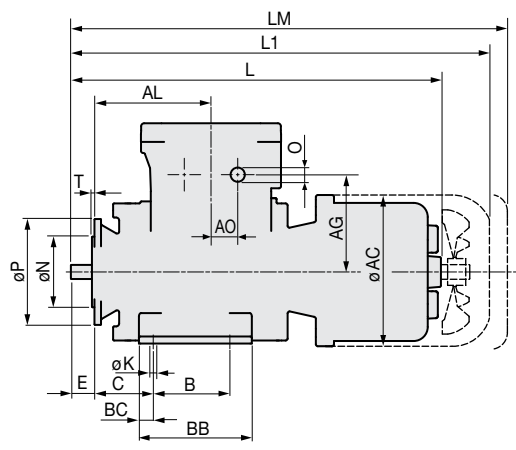
IM B34
