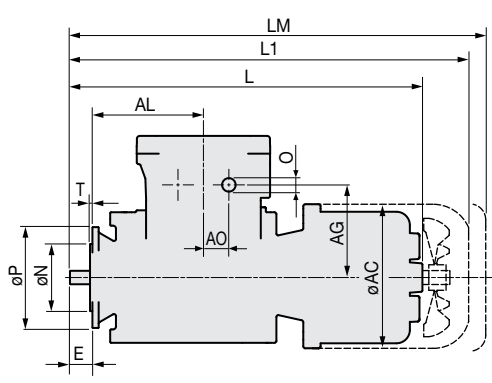
IM B14
