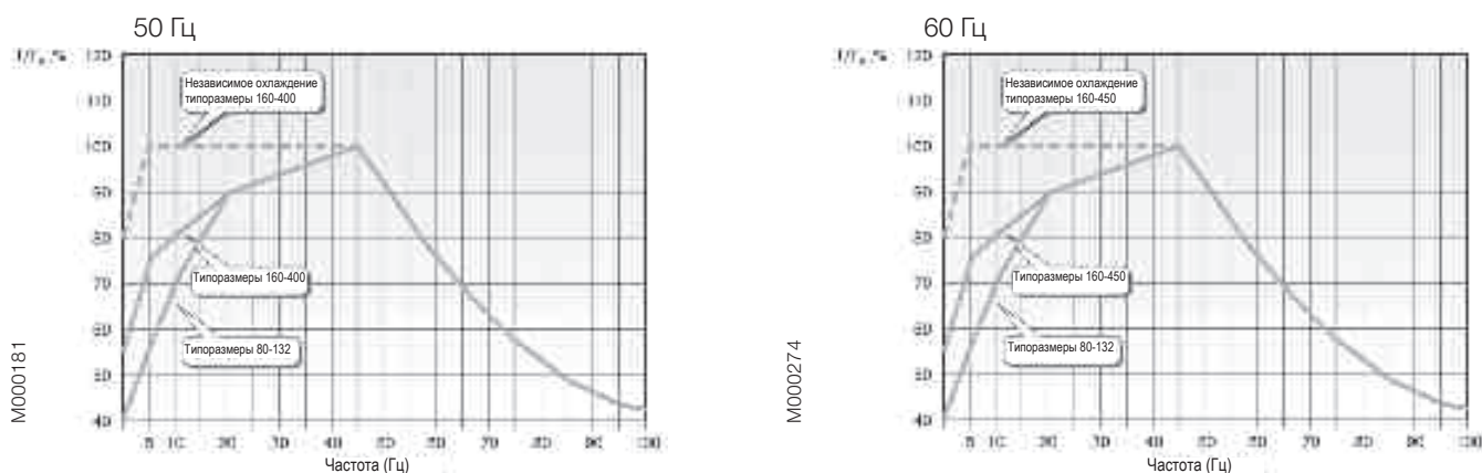
Рис. 3. Искробезопасные двигатели Ex nA, двигатели в чугунных и алюминиевых корпусах с защитой от воспламенения горячей пыли (DIP/Ex tD T125°C), номинальная частота двигателя 50/60 Гц
