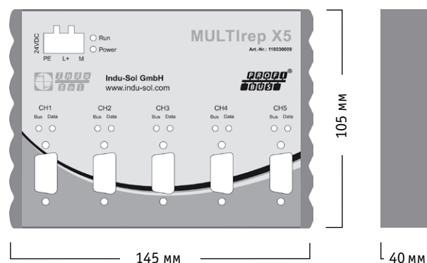
Рабочий чертеж
