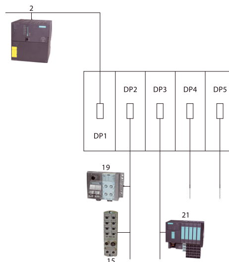
Пример соединения
