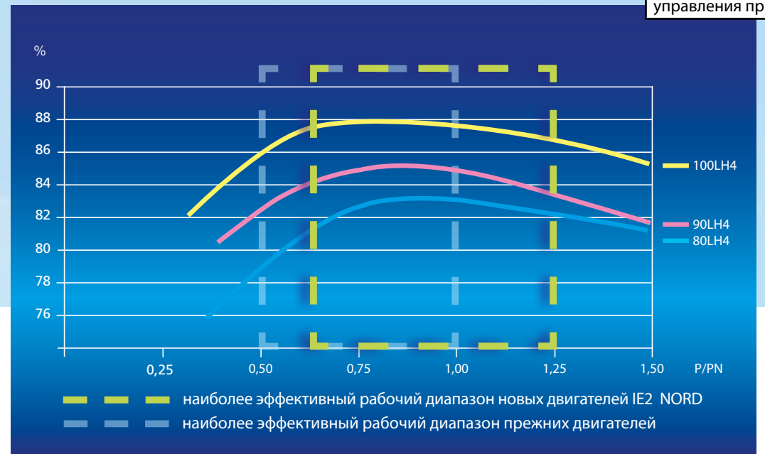
Графики демонстрируют принципиальные характеристики КПД асинхронных двигателей габаритов 100 LH4, 90 LH4 и 80 LH4.
