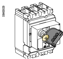
Блокировка поворотной рукоятки навесными замками или встроенным замком
