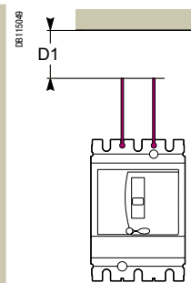
Аппараты с разделителями полюсов или длинной клеммной заглушкой
