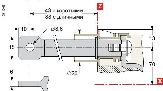
NSX100 - 250
