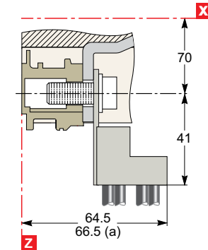
NSX100 - 250
