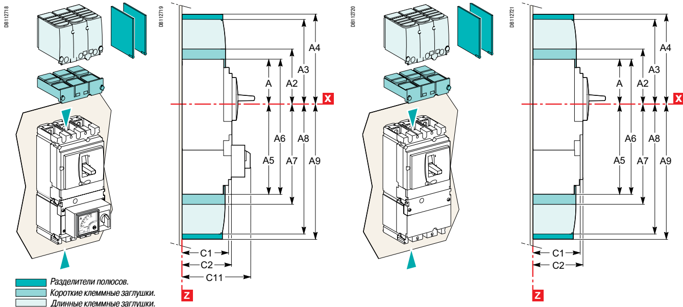
NSX100 - 250
