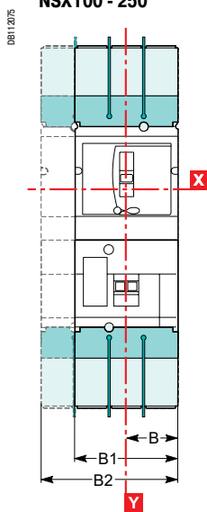
NSX100 - 250
