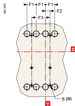
NSX100 - 630
