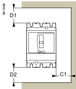
Аппарат без аксессуаров
