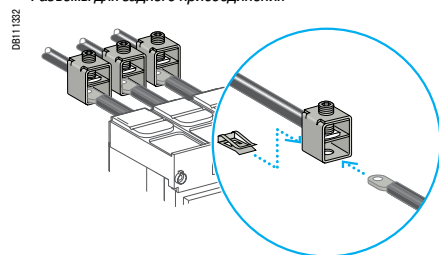
Присоединение кабелей без наконечников к NSX100 - 250
