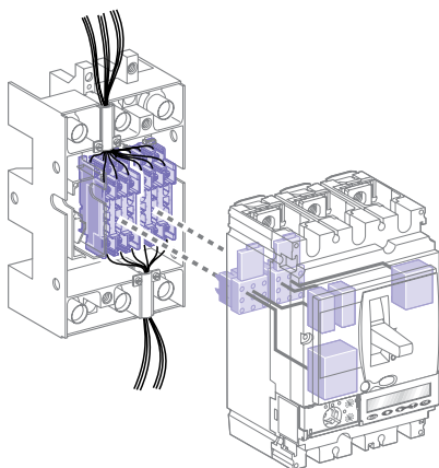
Втычной/выдвижной аппарат Compact NSX
