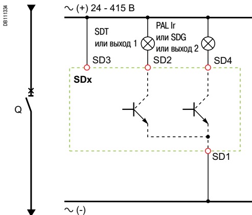
Электромотажная схема модуля SDx
