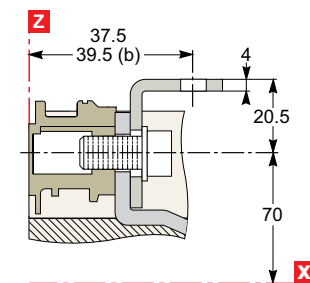
NSX100 - 250
