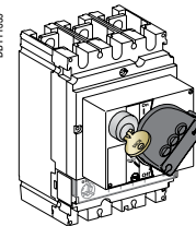
Блокировка поворотной рукоятки навесным или встроенным замком
