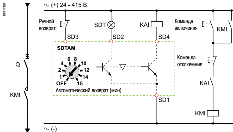
Электромотажная схема модуля SDTAM с функцией управления контактором
