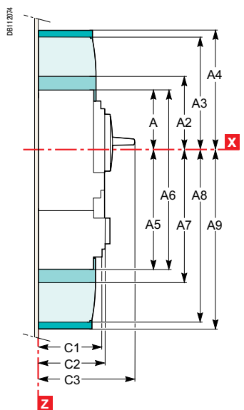
NSX100 - 250
