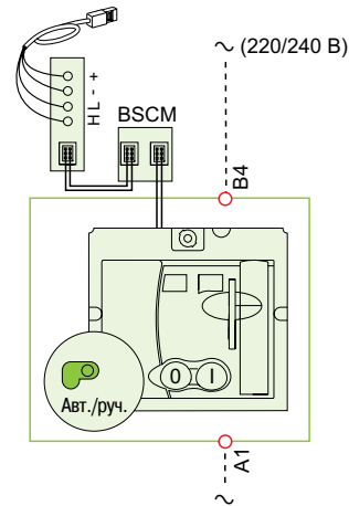
Коммутационный мотор-редуктор (MTc) (1)
