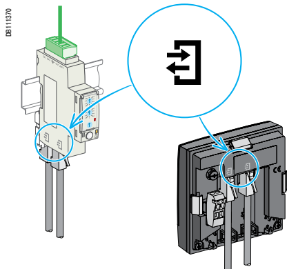
Символ присоединения совместимых модулей Compact NSX
