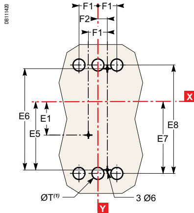
NSX100 - 250
