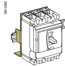
Крепление на DIN-рейке при помощи переходника
