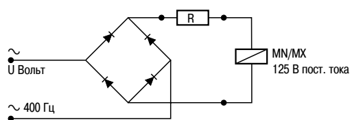
Схема подключения
