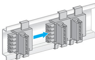
Монтаж при помощи аксессуаров для присоединения
