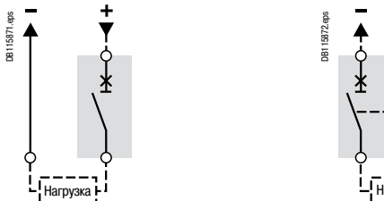
Выбор 1: стационарный 1-полюсный аппарат Compact NSX160N DC
