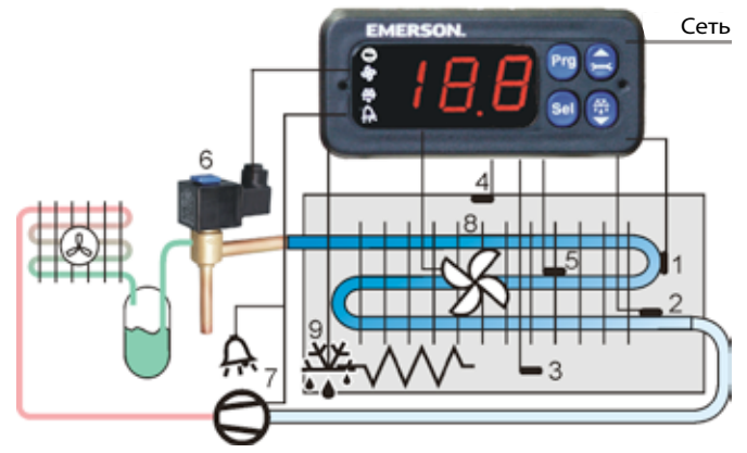
Контроллер торгового оборудования EC2-31x / -39x (EX2, темп./темп.)
